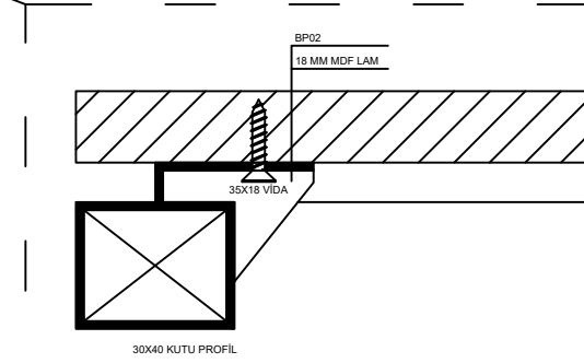
DETAY
