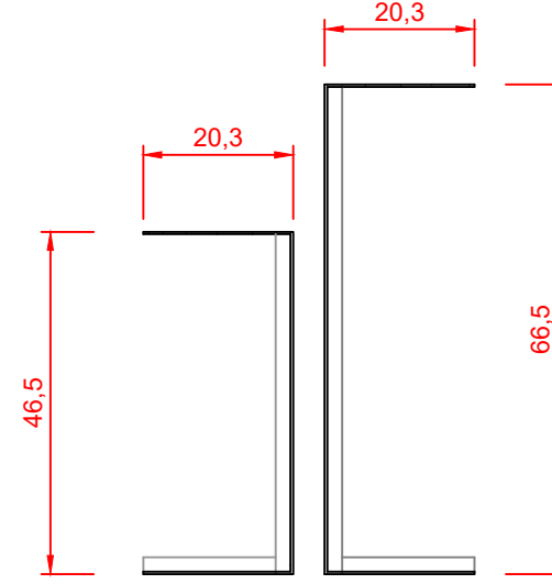
SAĞ YAN GÖRÜNÜŞ
