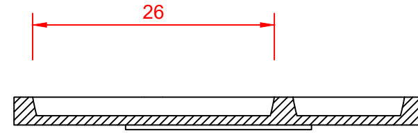
BB' KESİTİ
