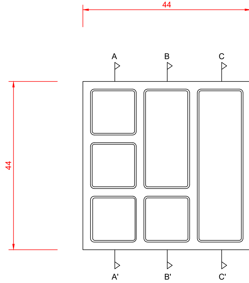
PLAN GÖRÜNÜŞ
