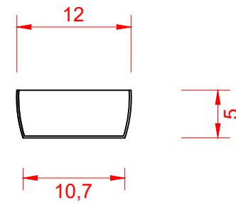
CC' KESİTİ
