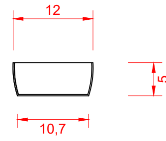
CC' KESİTİ
